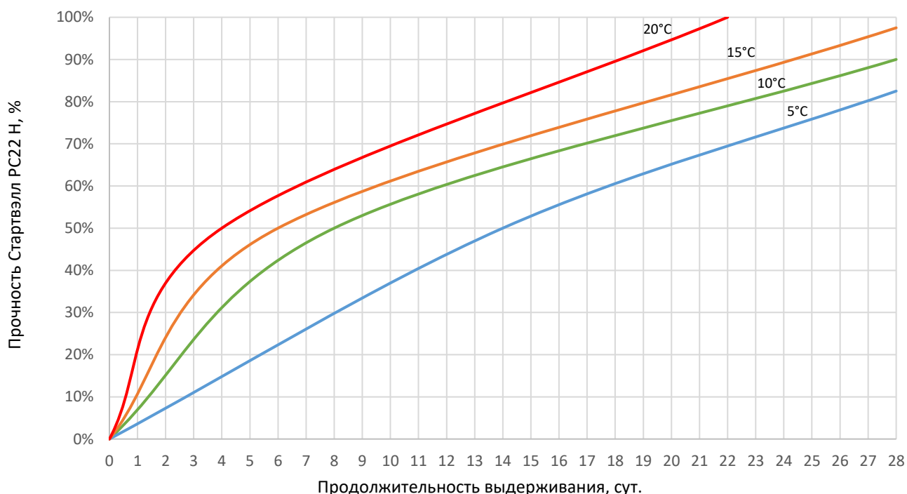
Рис.1. Прочность цементной штукатурки серияPRO в зависимости от температуры и продолжительности выдерживания.
