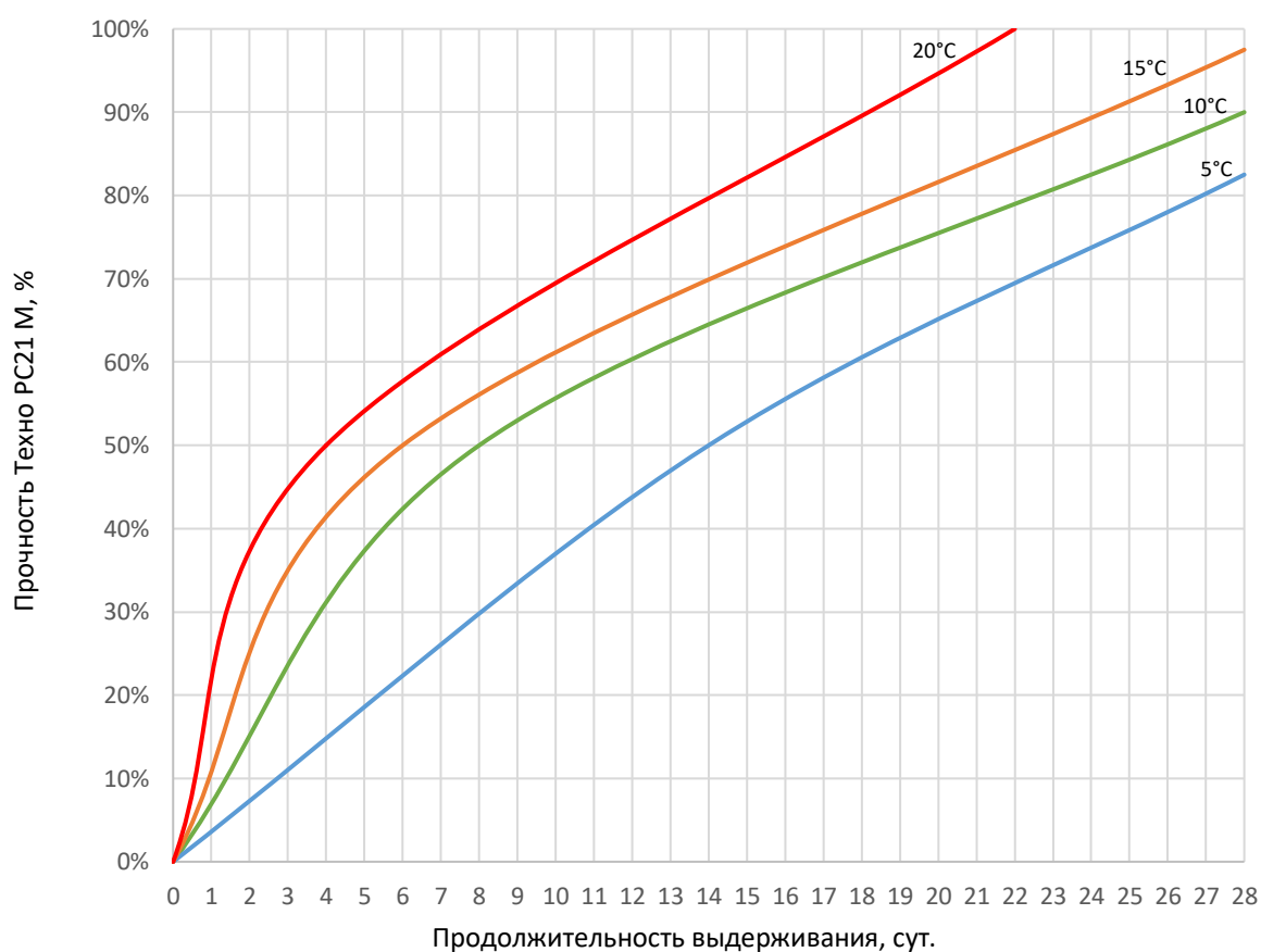
Рис.1. Прочность цементной штукатурки Техно РС21/2 MF в зависимости от температуры и продолжительности выдерживания.
