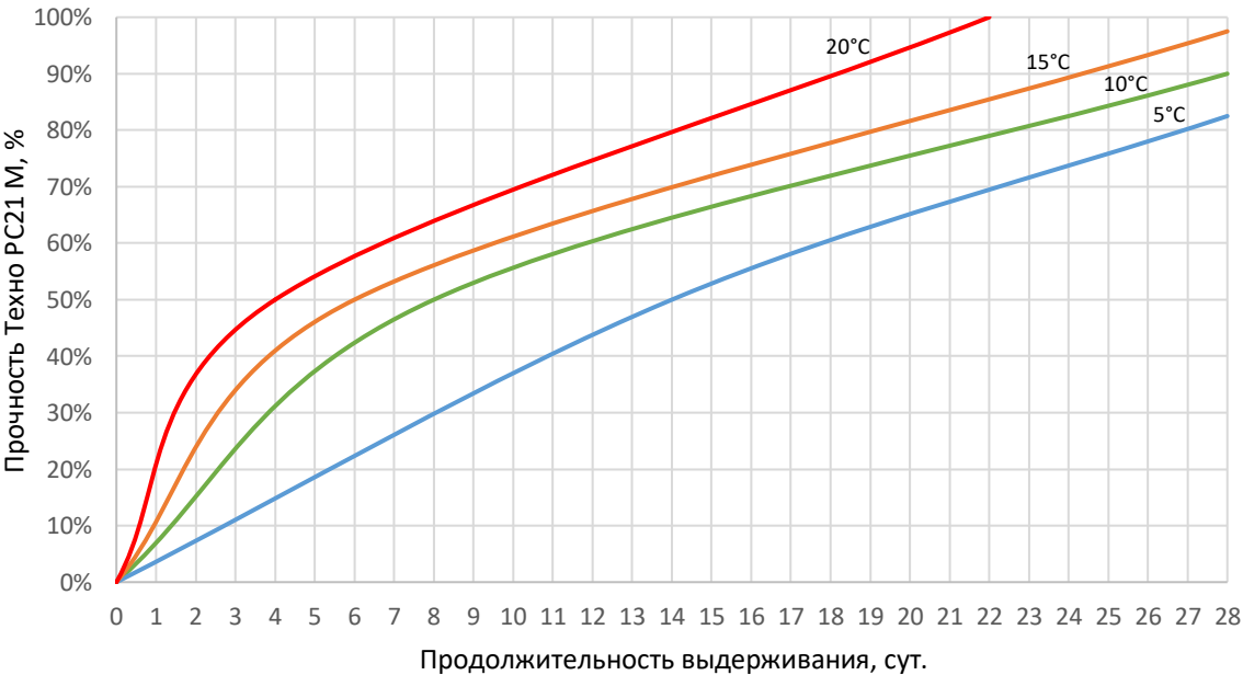
Рис.1. Прочность цементной штукатурки Техно PC21 М в зависимости от температуры и продолжительности выдерживания.
