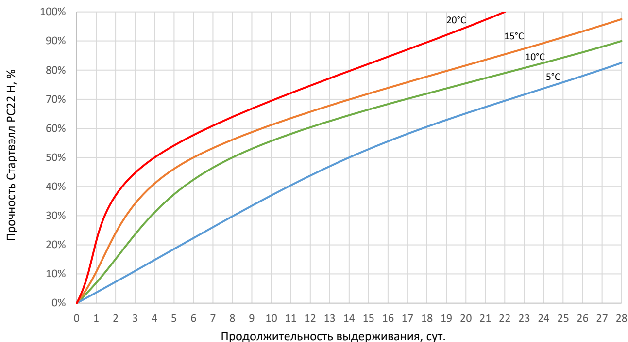
Рис.1. Прочность цементной штукатурки Стартвэлл РС22 Н в зависимости от температуры и продолжительности выдерживания.
