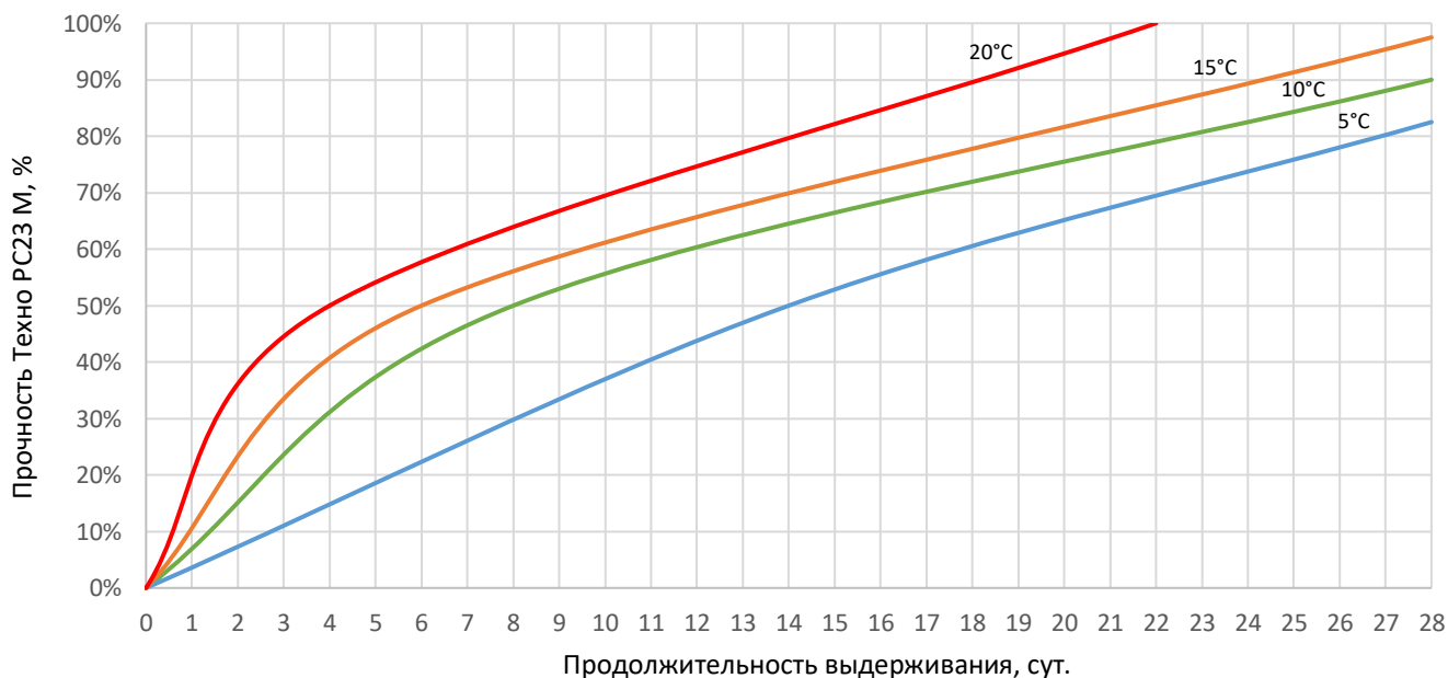
Рис.1. Прочность цементной штукатурки шпаклевки Техно PC23 М в зависимости от температуры и продолжительности выдерживания.
